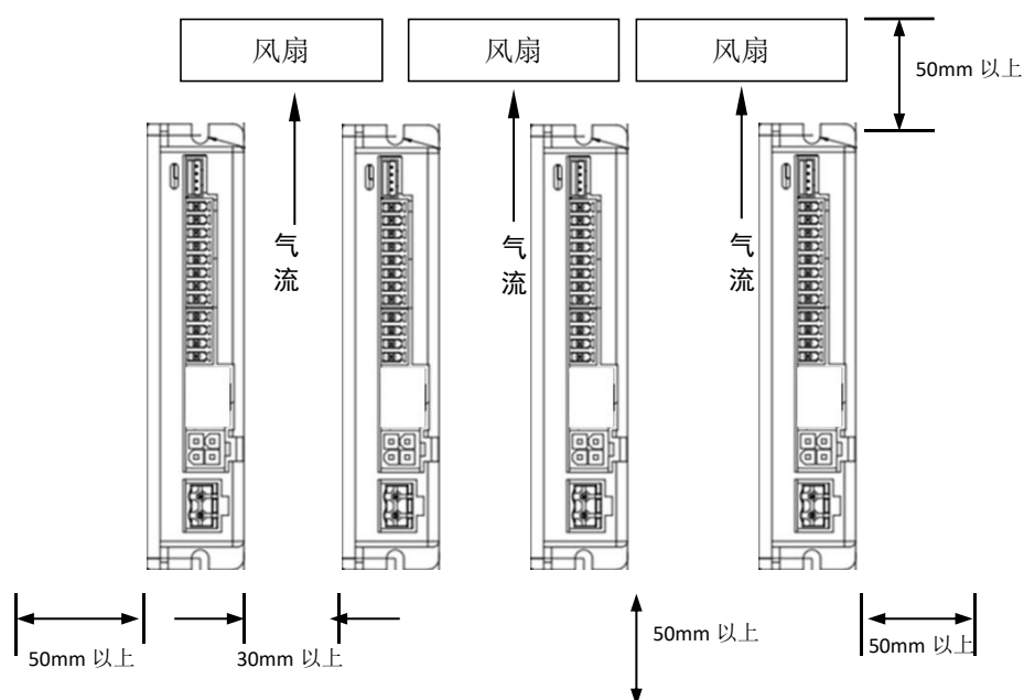
图 2-3 驱动器安装间隔示意图
